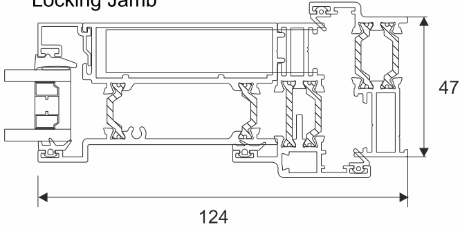
Locking Jamb
